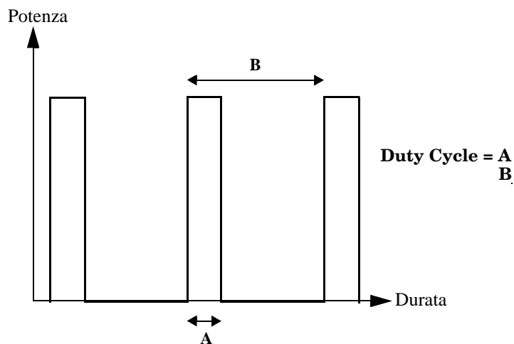
Figura 2-10: Segnale ad impulsi
