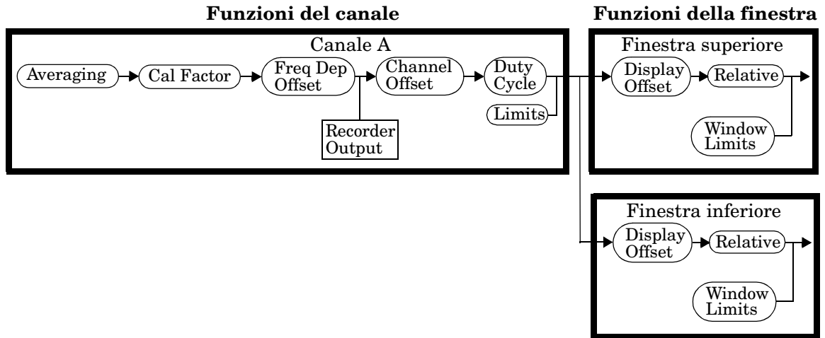
Figura 2-22: Come vengono calcolate le misure
