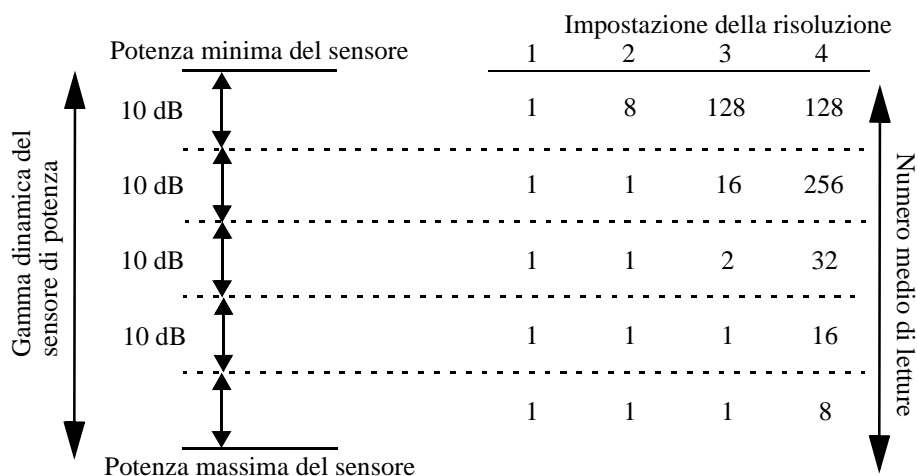
Figura 2-9: Letture medie
