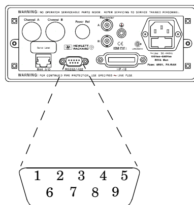
Figura 2-18: Distribuzione dei pin in RS232/422
