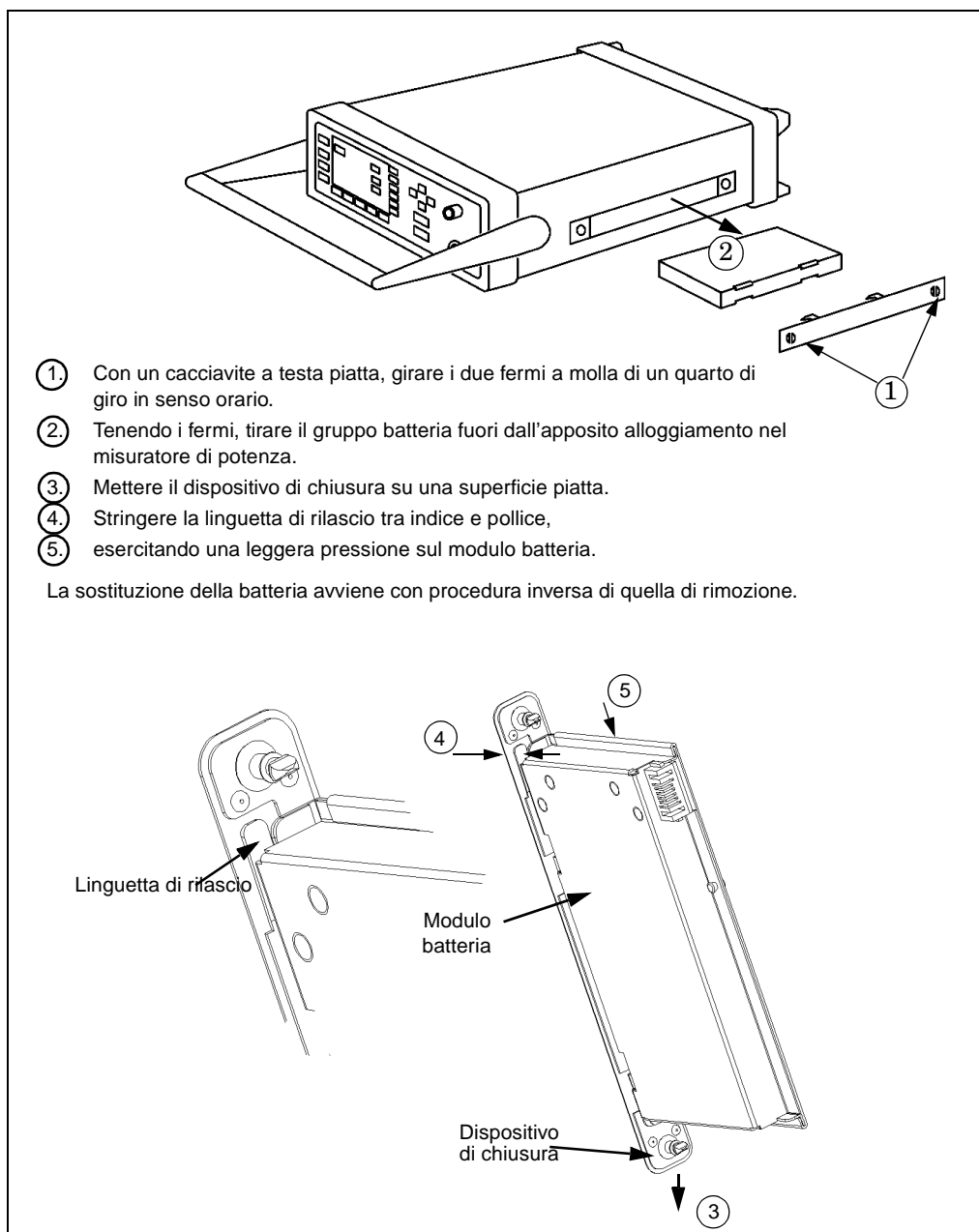
Figura 2-2: Rimozione/Sostituzione della batteria
