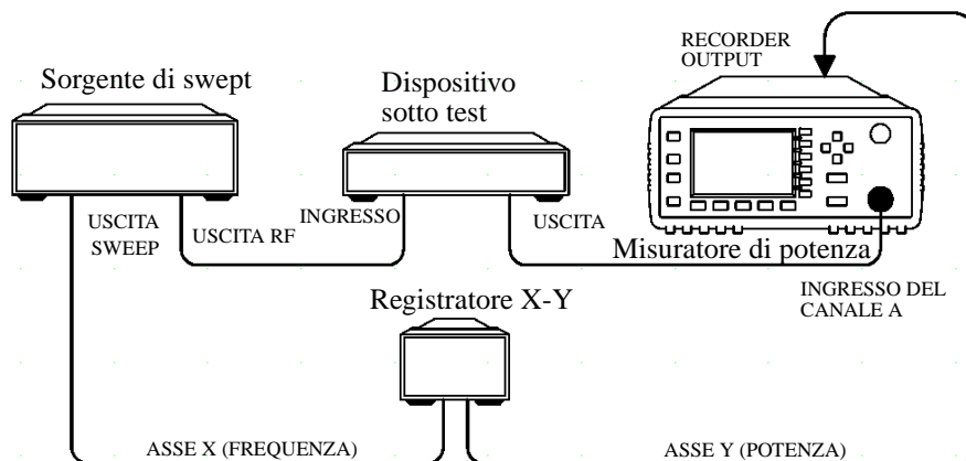
Figura 2-20: Impostazione test per registrare le misure di swept
