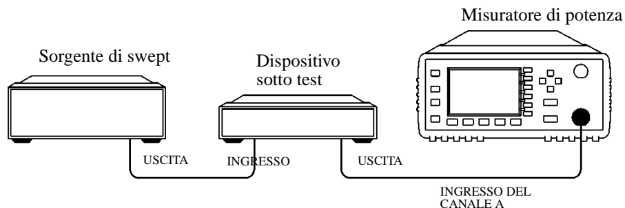
Figura 2-11: Applicazione del controllo dei limiti
