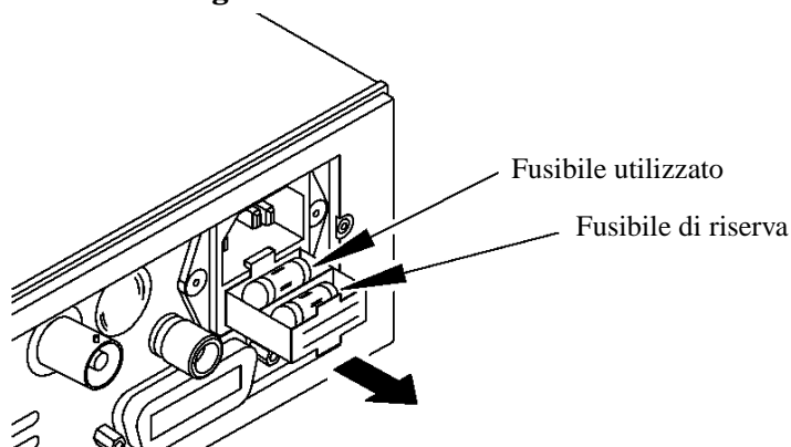
Figura 2-23: Sostituzione del fusibile
